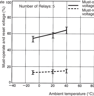
G2A-434A DC
