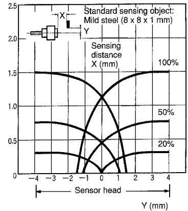
E2C-X1R5AH + E2C-JC4CH
