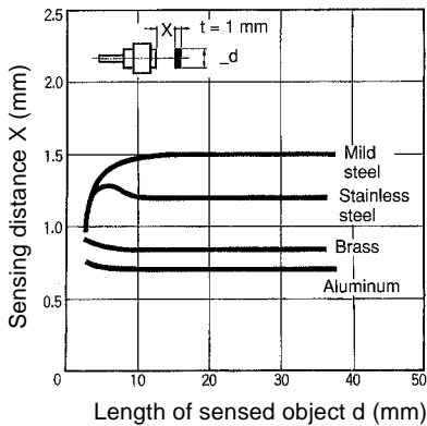
E2C-X1R5AH + E2C-JC4CH
