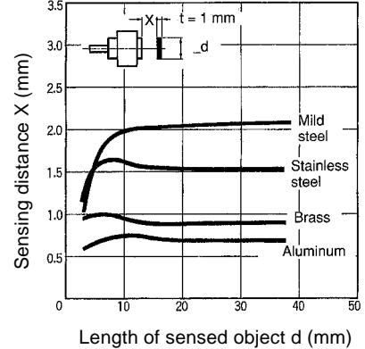
E2C-X2AH + E2C-JC4DH
