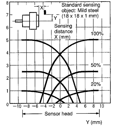
E2C-X5AH + E2C-JC4EH
