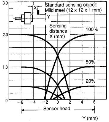
E2C-X2AH + E2C-JC4DH
