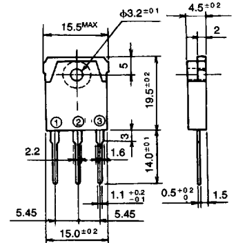
TO3P
