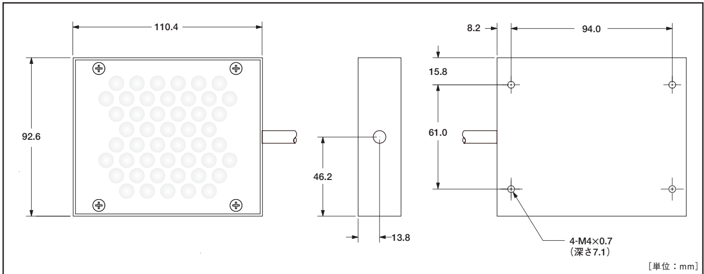
Fig.1 外形
