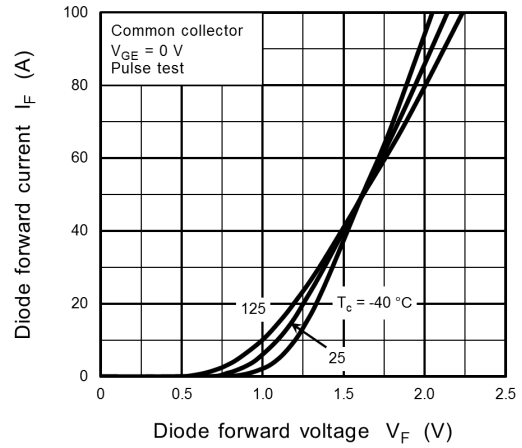
Fig. 8.14 I_F - V_F
