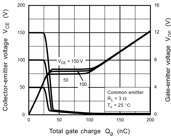
Fig. 8.9 V_{CE} , V_{GE} - Q_g
