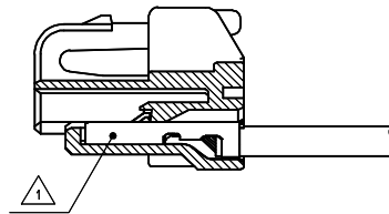
△1 ターミナル装着図 TERMINAL ASSEMBLY DRAWING
